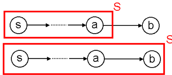
Figuur 2.5: De verzameling S groeit met de knoop b
