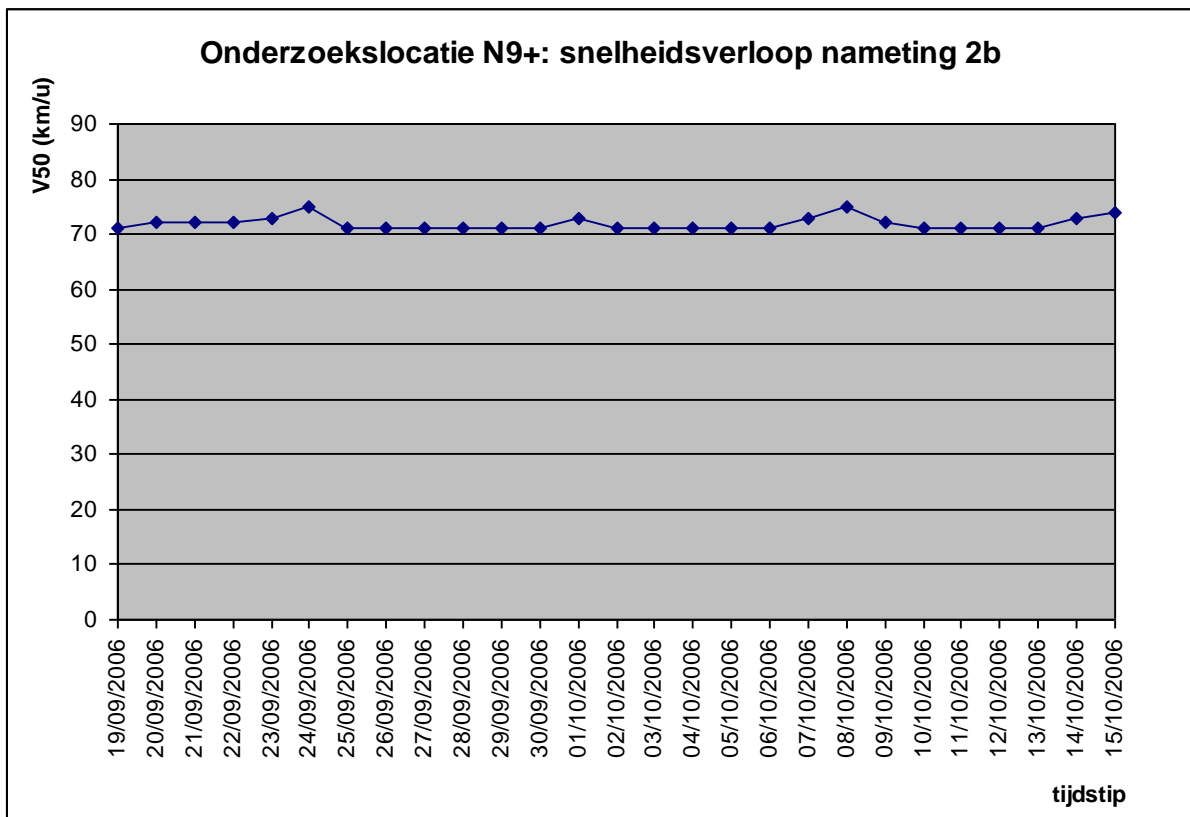
Figuur 19: snelheidverloop op onderzoekslocatie N9+ bij nameting 2b
