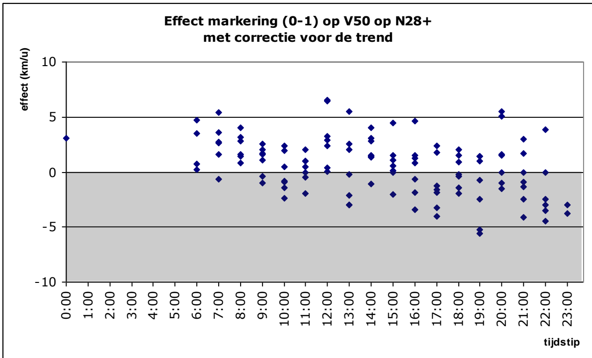
Figuur 5: effect van markering (effect 0-1) op N28, rijrichting + Berekende effectwaarden schommelen rond 0-waarde, met een maximumwaarde van +7 km/u en een minimumwaarde van -6 km/u.
