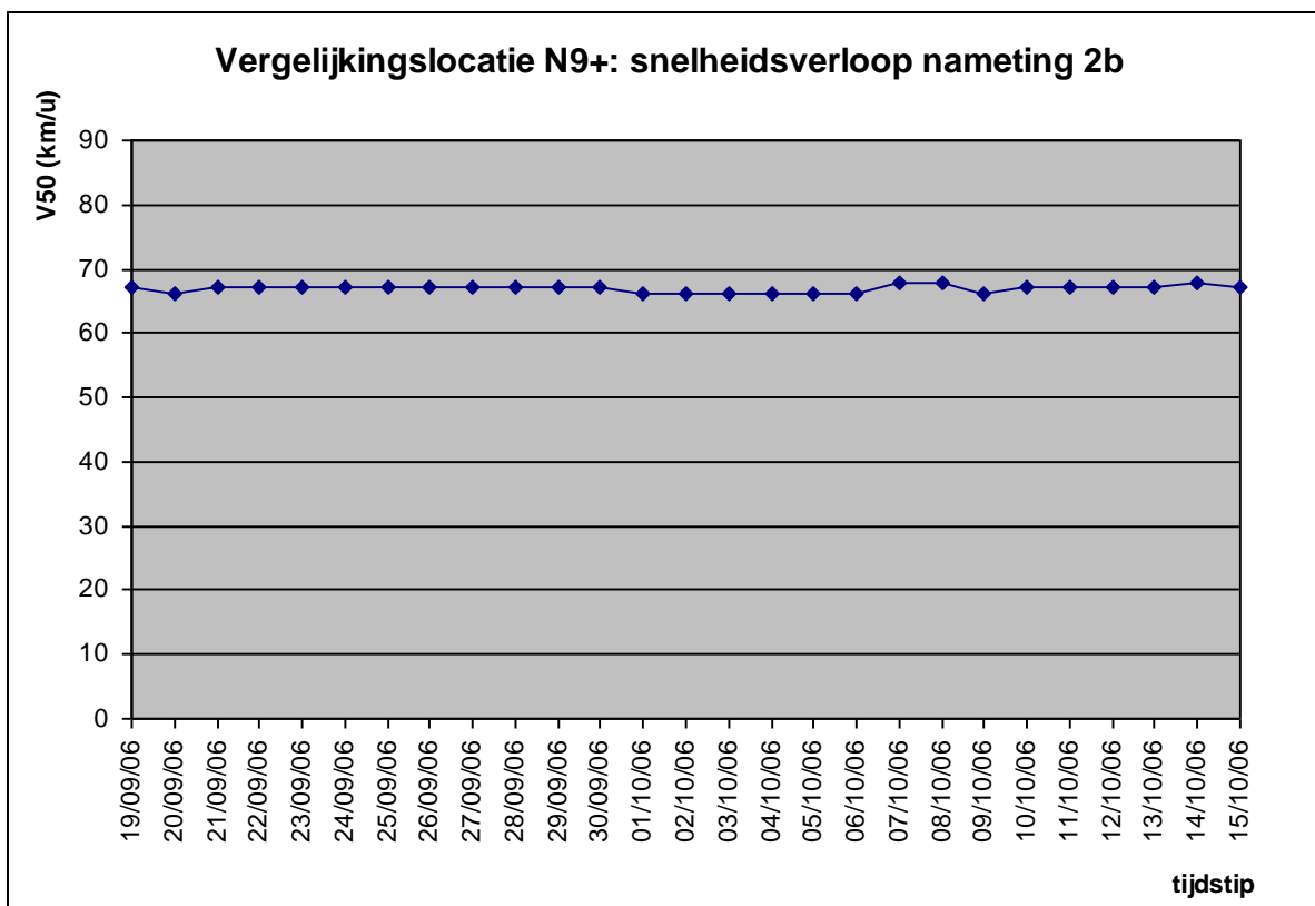
Figuur 25: snelheidverloop op vergelijkingslocatie N9+ bij nameting 2b
