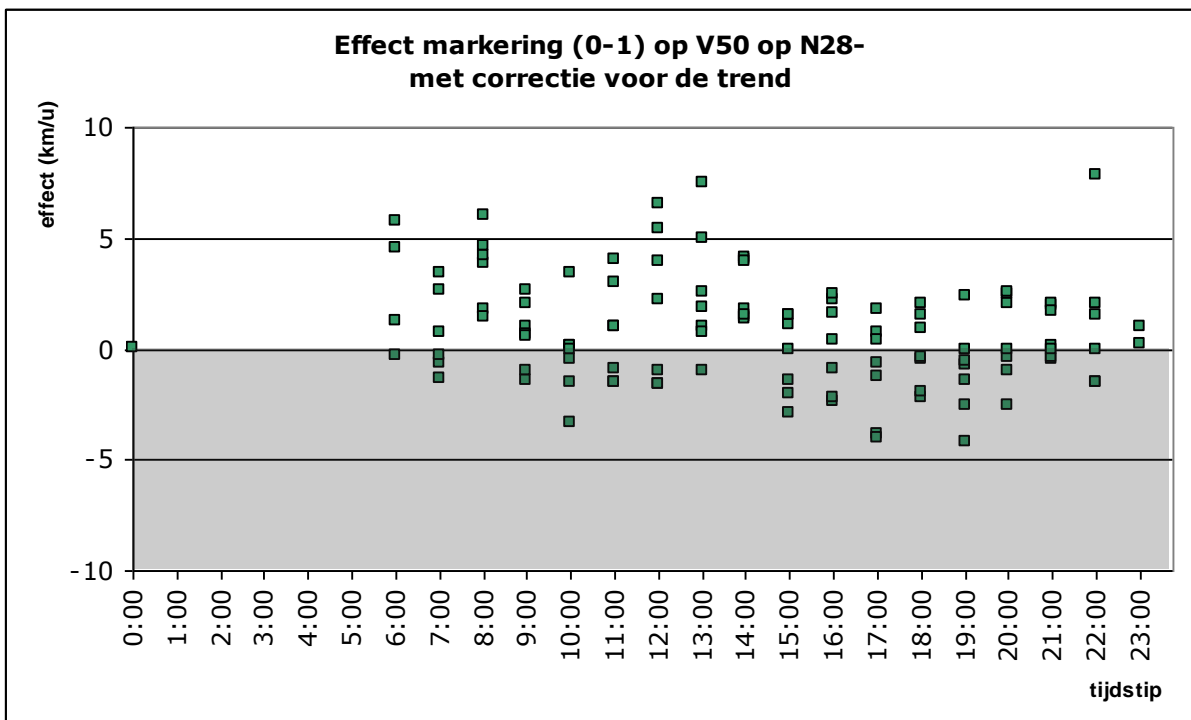
Figuur 6: effect markering (effect 0-1) op N28, rijrichting - Ook in de andere richting liggen alle waarden rond 0 km/u. Piekwaarden zijn een stijging van +8km/u en een daling van -4 km/u.
