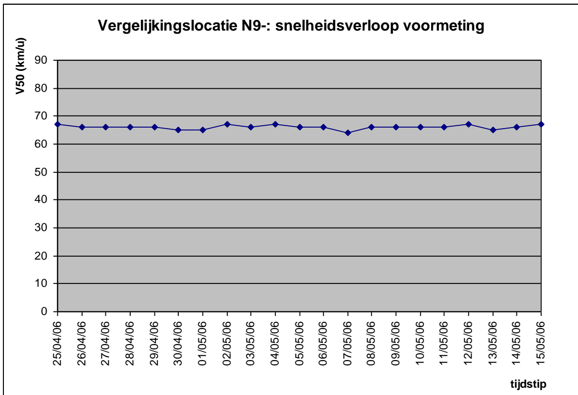
Figuur 20: snelheidverloop op vergelijkingslocatie N9- bij voormeting
