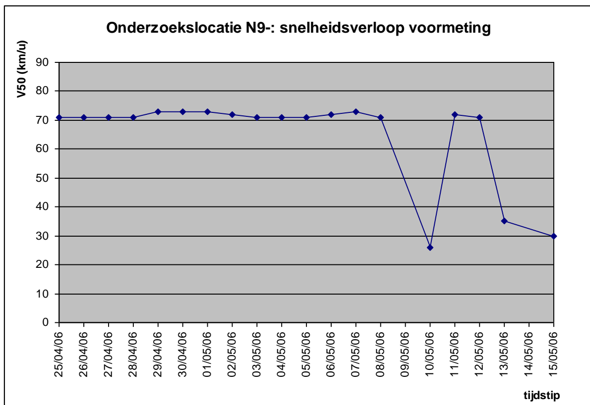
Figuur 15: snelheidsverloop op onderzoekslocatie N9- bij voormeting
