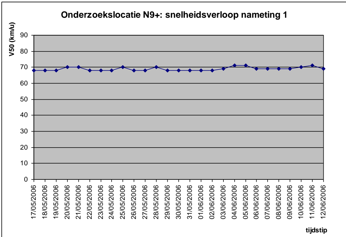
Figuur 17: snelheidverloop op onderzoekslocatie N9+ bij nameting 1
