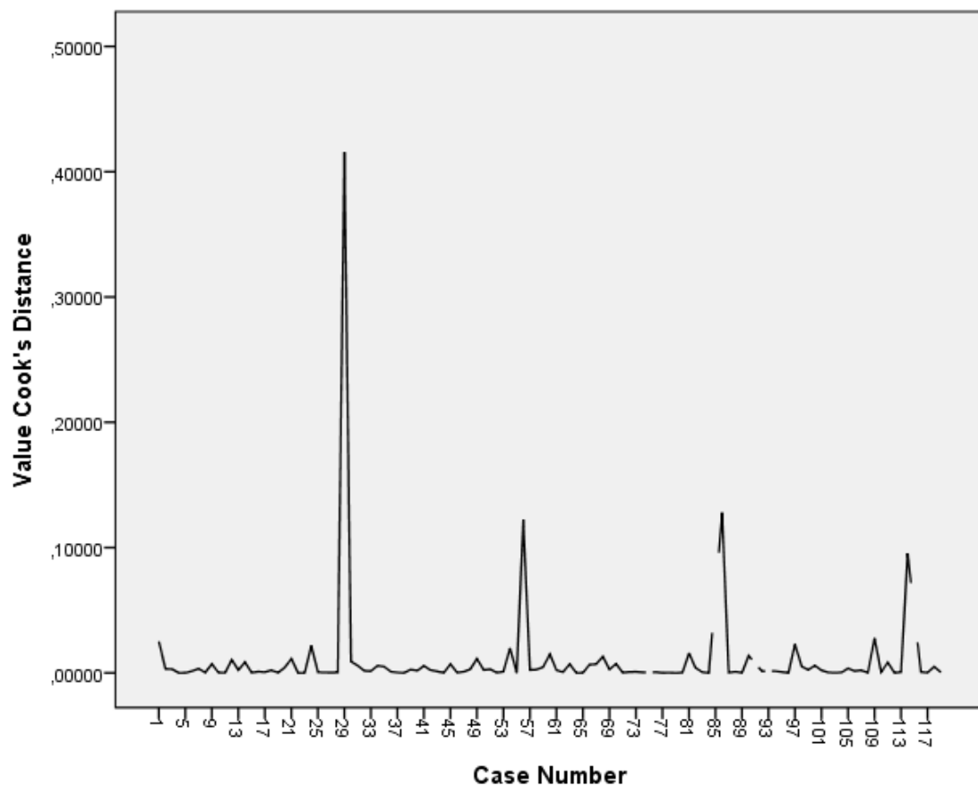
Figuur 17: Cook's Distance (Eigen onderzoek)
