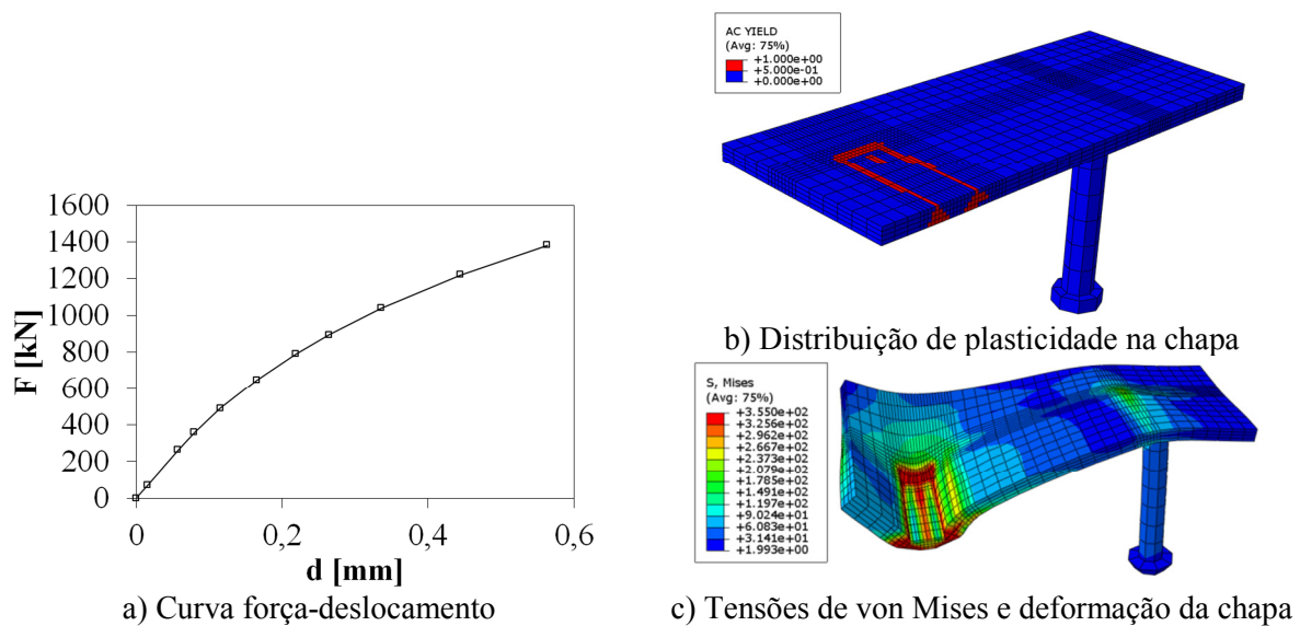
Fig. 3: Resultados do modelo numérico reproduzindo a chapa de ancoragem à compressão
