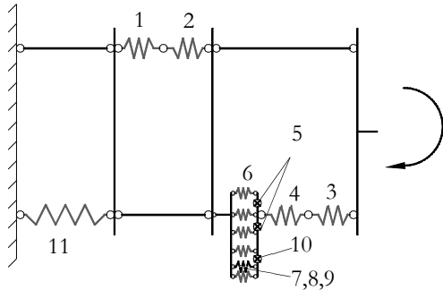
Fig. 12: Modelo de molas representativo da ligação entre viga mista e parede de betão armado
