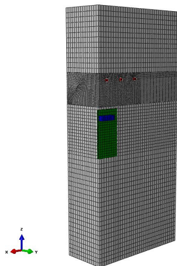
Fig. 6: Modelo para estudo da componente “JointLink”
