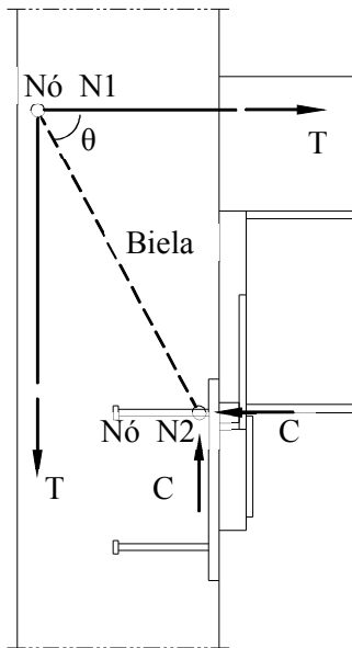
Fig. 8: Modelo de bielas e tirantes idealizado para a componente “JointLink”
