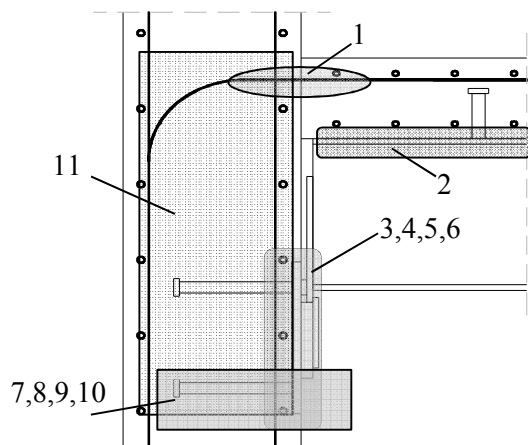
Fig. 1: Configuração da ligação entre viga mista e parede de betão armado em estudo
