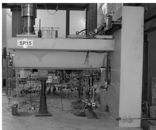
Fig. 10: Esquema de ensaio da ligação entre viga mista e parede de betão armado [5]
