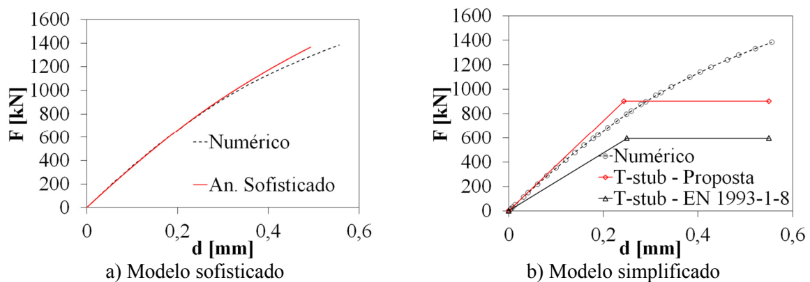
Fig. 5: Aplicação e comparação dos modelos analíticos
