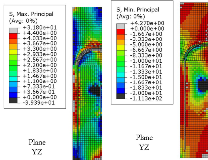
Fig. 7: Tensões principais máximas e mínimas na parede de betão armado
