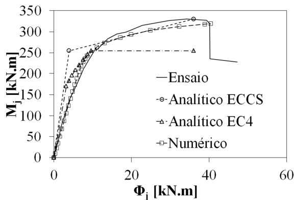
Fig. 14: Comparação das curvas momento-rotação obtidas pela via experimental, numérica e analítica
