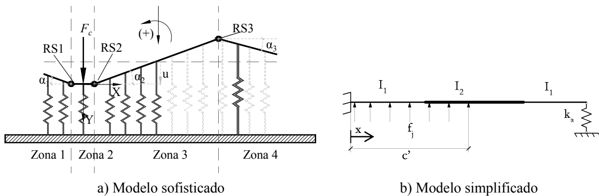
Fig. 4: Modelos analíticos para a chapa de ancoragem à compressão
