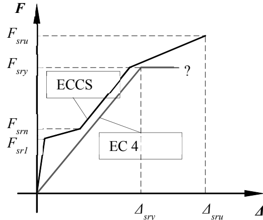
Fig. 13: Curvas força-deslocamento representativas dos modelos usados para caracterizar a componente 1
