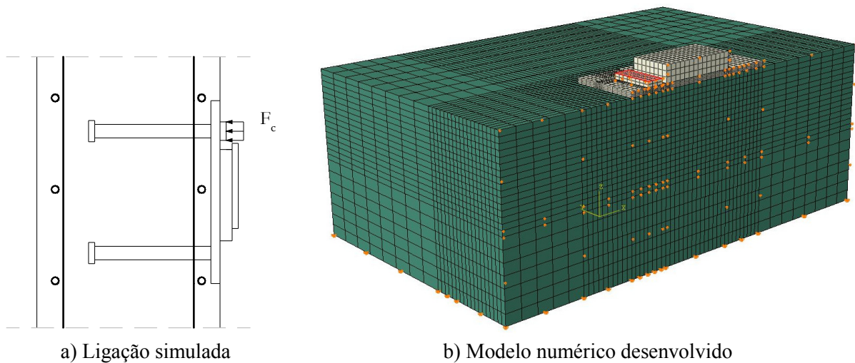
Fig. 2: Chapa de ancoragem submetida a compressão
