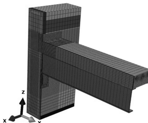
Fig. 11: Modelo numérico desenvolvido para reproduzir o comportamento da ligação entre viga mista e parede de betão armado
