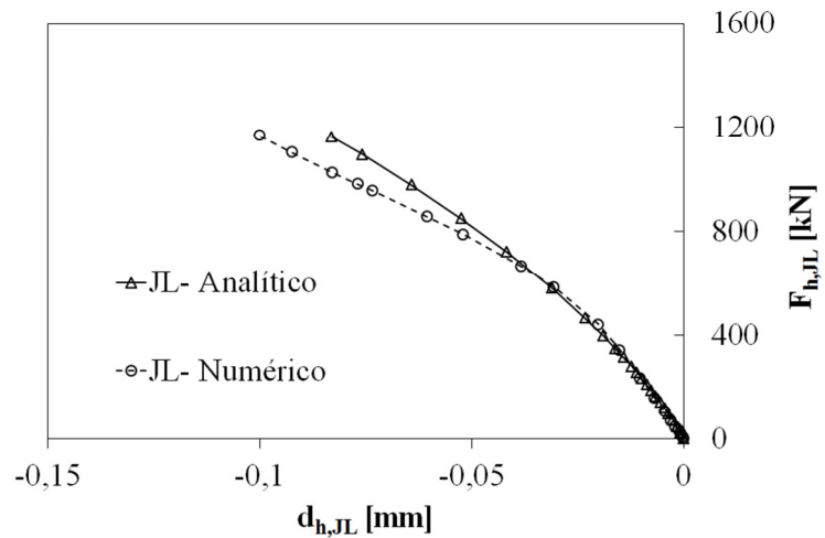
Fig. 9: Resultado de aplicação do modelo analítico e comparação com o resultado do modelo numérico
