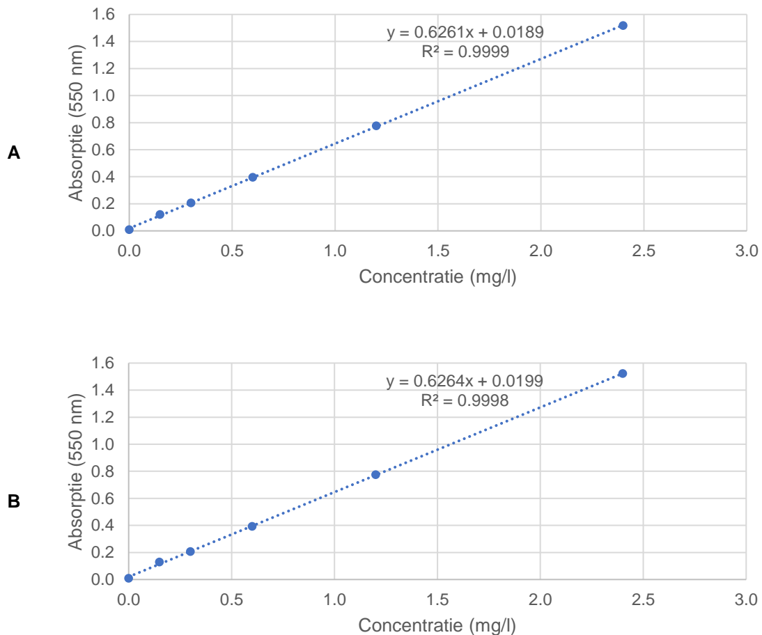
Figuur 16: (A) Kalibratielij van NaNO 2 na 10 minuten (B) en na 30 minuten (550 nm).
