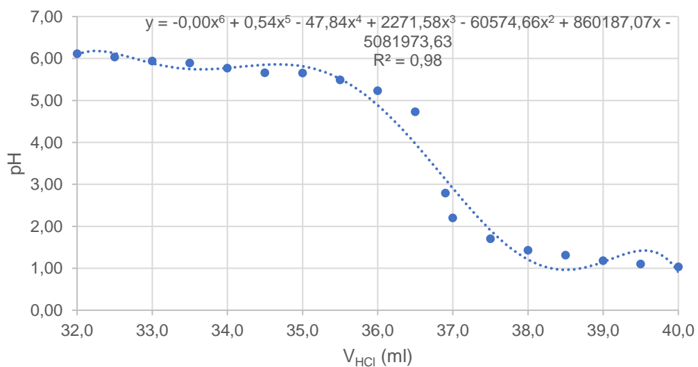
Figuur 12: Curvefitting van de beperkte dataset rond equivalentiepunt drie van Titratie 3.
