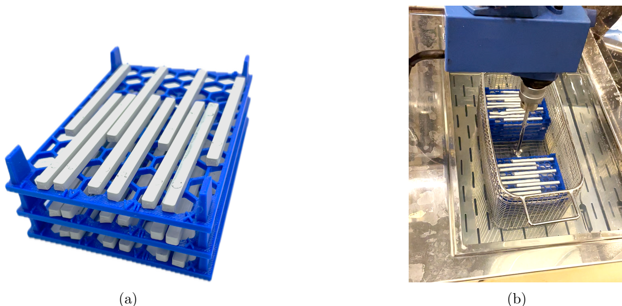
Figuur 3.6: (a) Rekjes met spuitgietsproducten voor water ontbinden; (b) Opstelling ontbindingsproces
