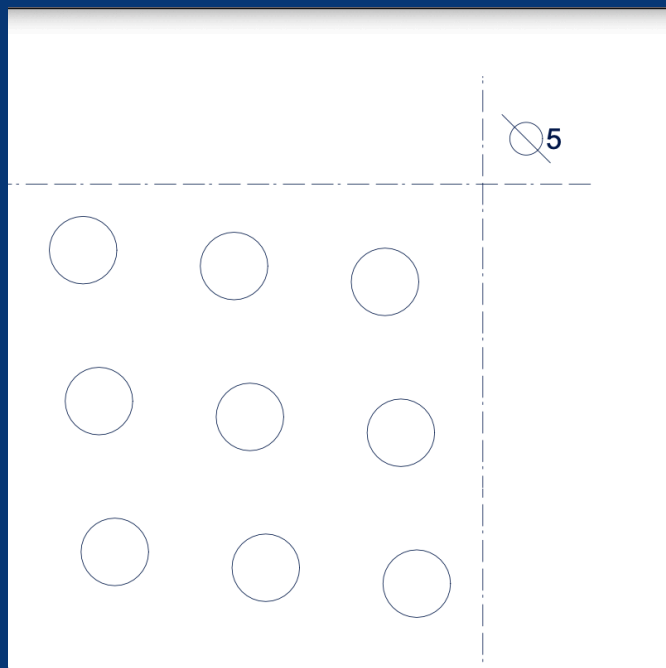
Detail geperforeerde plaat, 2025
