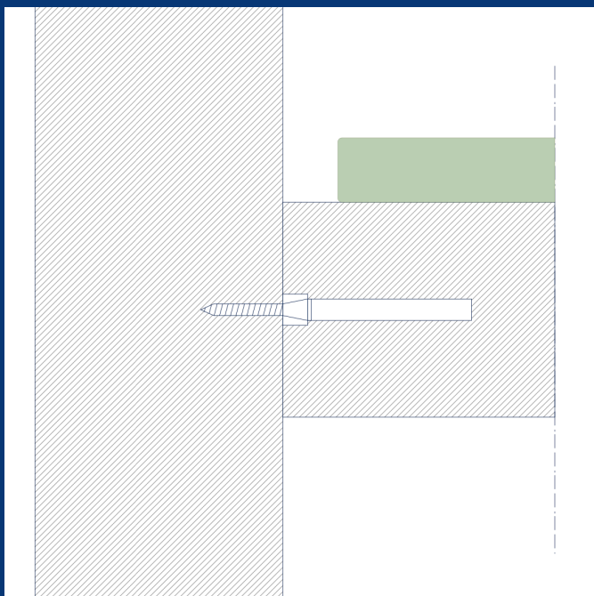
Detail verankering muur, 2025
