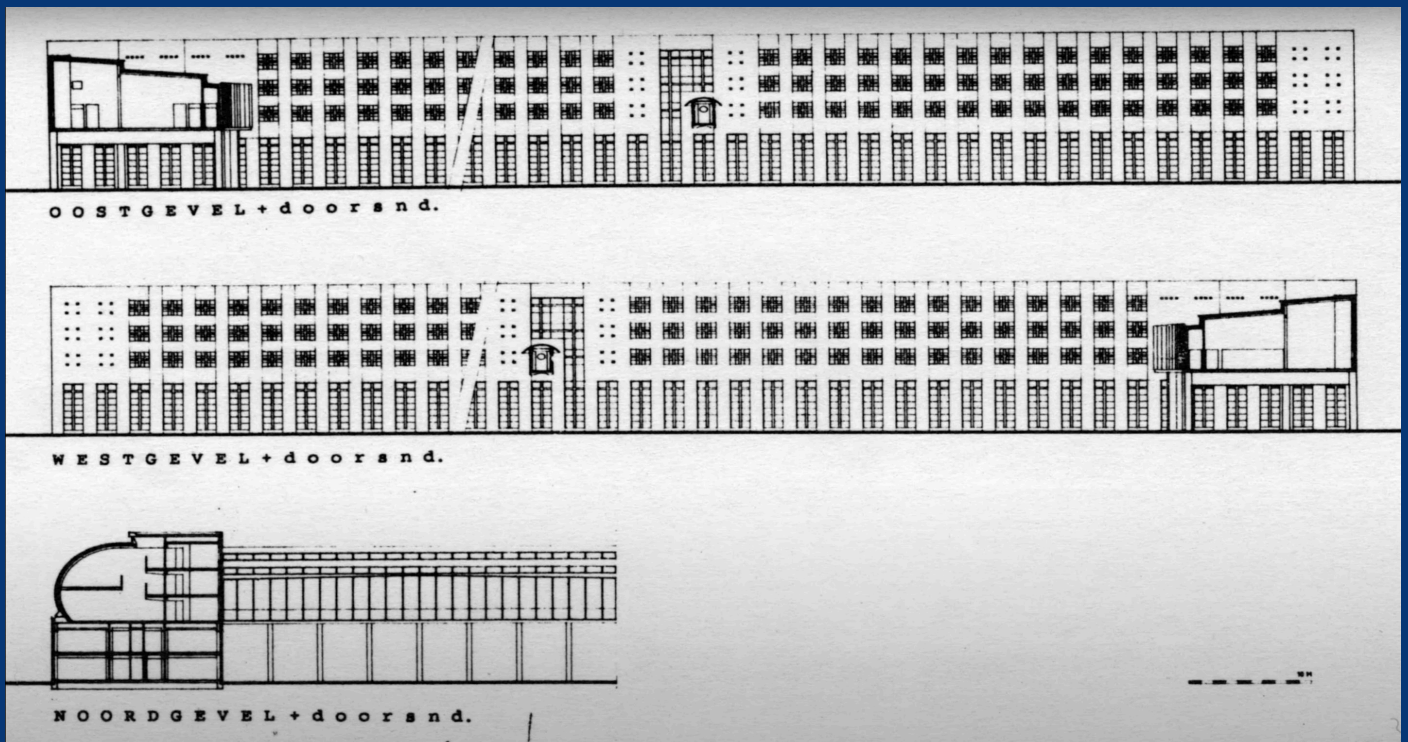
Afbeelding 4: Gevelplannen gevangenis in Zwaag, 1987
